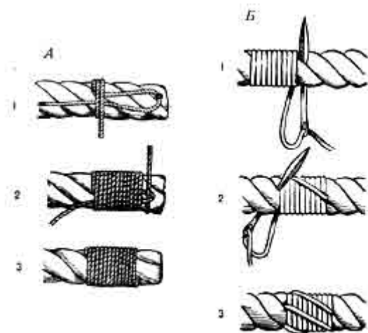
Рис. 56. Марки: А — простая, Б — прошивная
