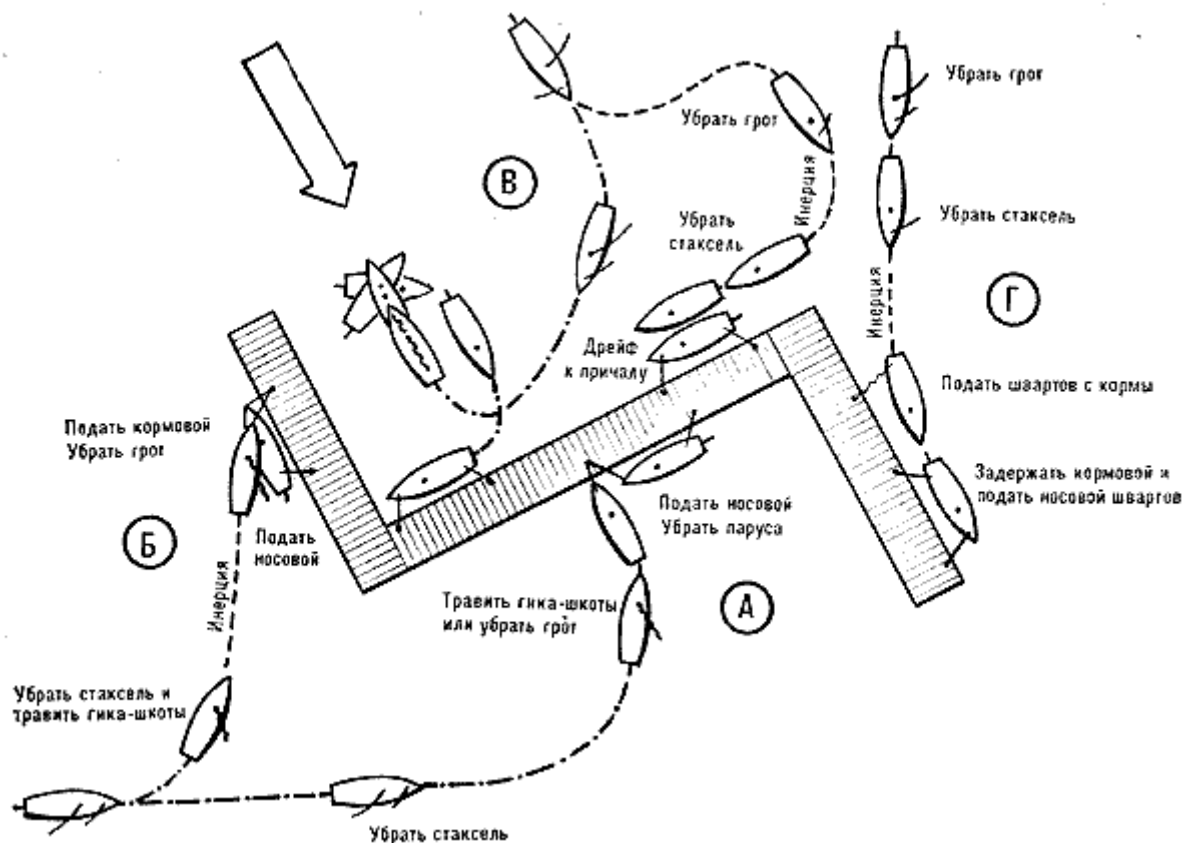
Рис. 125. Как подойти к причалу:
