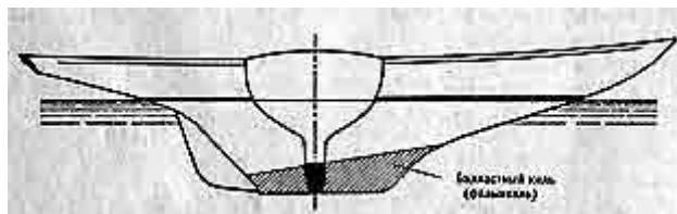
Рис. 4. Килевая яхта
