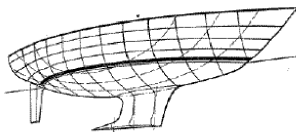
Рис. 86. Линии теоретического чертежа на корпусе яхты
