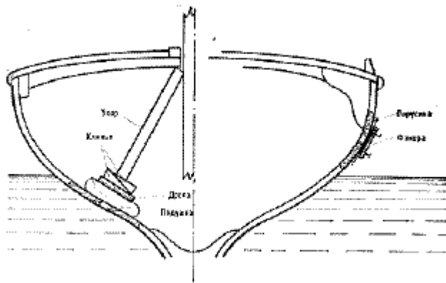
Рис. 136. Заделка надводной и подводной пробоины
