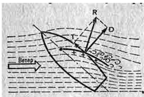
Рис. 3. Действие ветра на паруса яхты, идущей под острым углом к ветру
