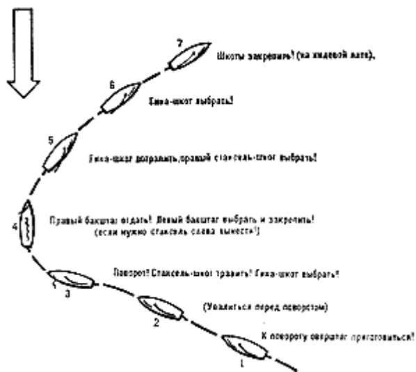
Рис. 108. Поворот оверштаг
