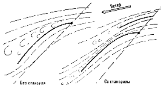
Рис. 97. Работа стакселя
