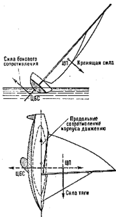
Рис. 100. Влияние крена на приведение яхты к ветру
