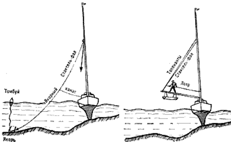
Рис. 139 Способы закрепления яхты на мели
