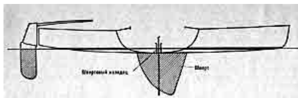
Рис. 5. Швертбот
