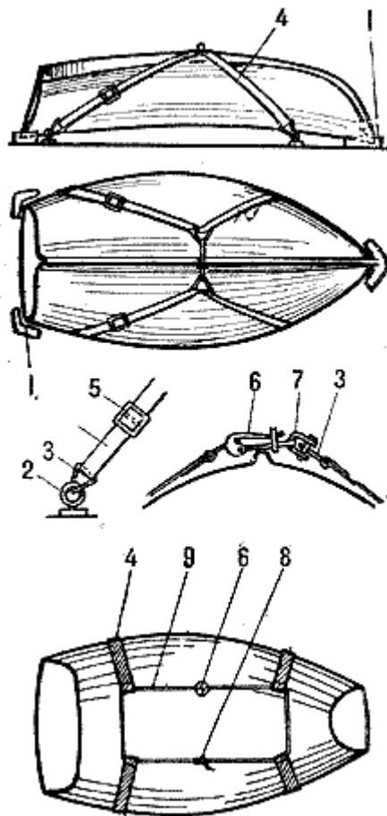
Рис. 132. Два способа крепления тузика по-походному:
