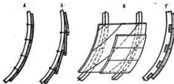
Рис. 29. Виды обшивки:
