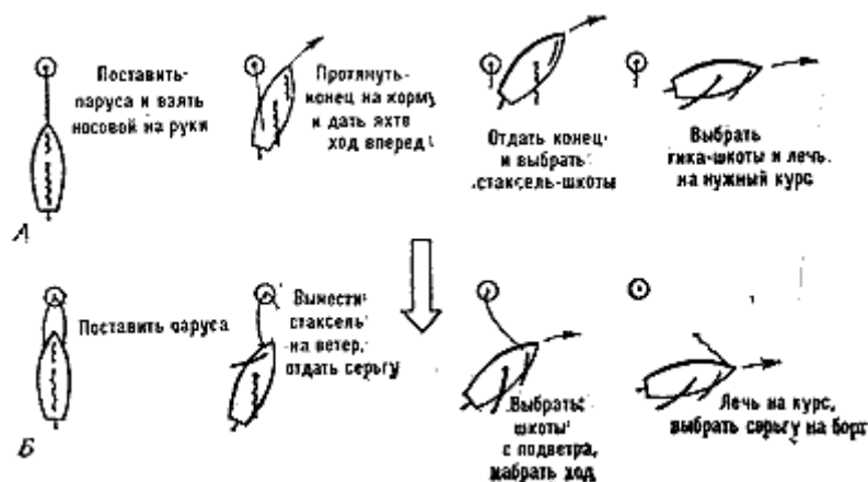
Рис. 122. Отход от буя или бочки А. — если яхта стояла на носовом, закрепленном на бочке, конце; Б — если яхта стояла на носовом конце, заложеном серьгой
