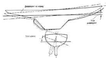
Рис. 77. Крен и дифферент
