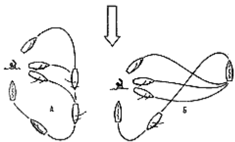
Рис. 134 Подход к упавшему за борт на курсах бейдевинд — крутой бакштаг:
