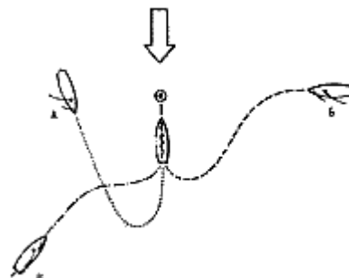
Рис. 128. Схема подхода к якорной стоянке или бочке
