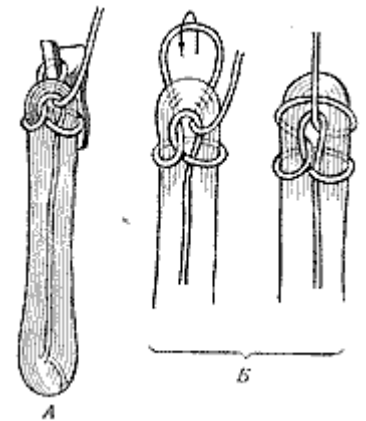
Рис. 103. Фал в походной бухте
