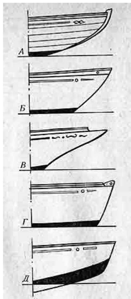
Рис. 11. Формы носовых частей:
