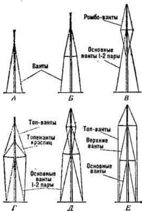
Рис. 38. Проводка вант:
