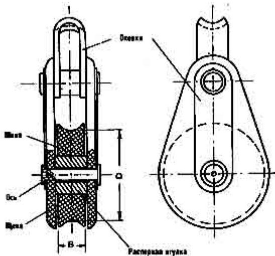
Рис. 45. Пластмассовый блок и его части
