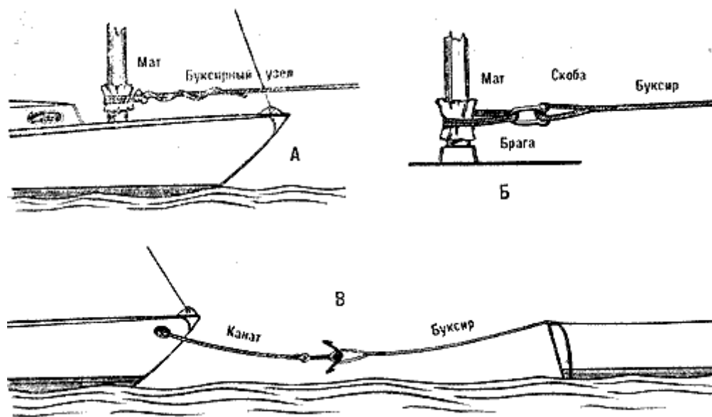
Рис. 137. Способы крепления буксира:
