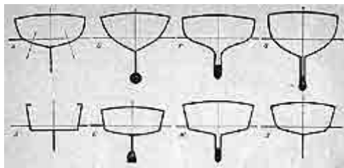
Рис. 9. Формы мидель-шпангоутов.
