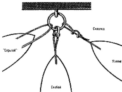
Рис. 130. Способы крепления швартовов за рым
