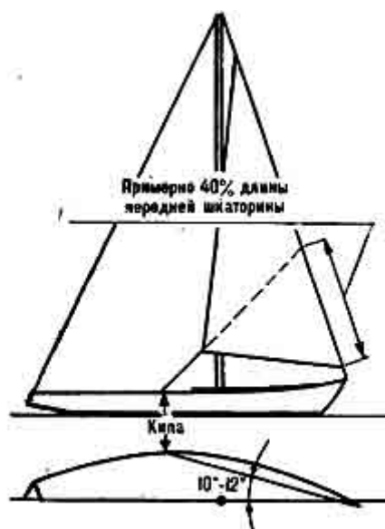
Рис. 46. Проводка стаксель-шкотов
