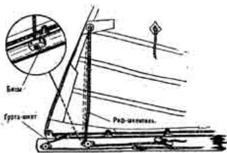
Рис. 42. Нок гика
