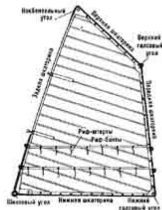
Рис. 36. Гафельный грот и его части
