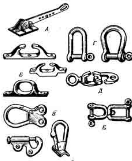
Рис. 51. Дельные вещи:
