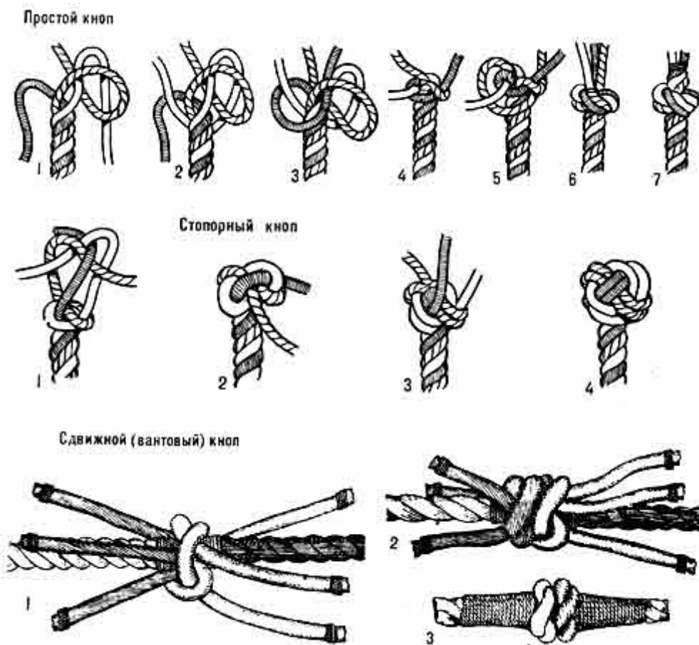
Рис. 69. Кнопы
