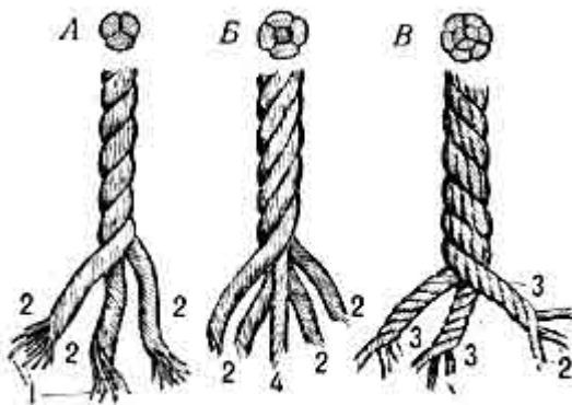
Рис. 55. Растительные тросы:
