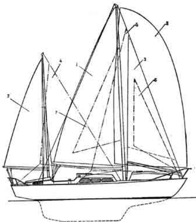
Рис. 34. Парусность бермудского кэча:
