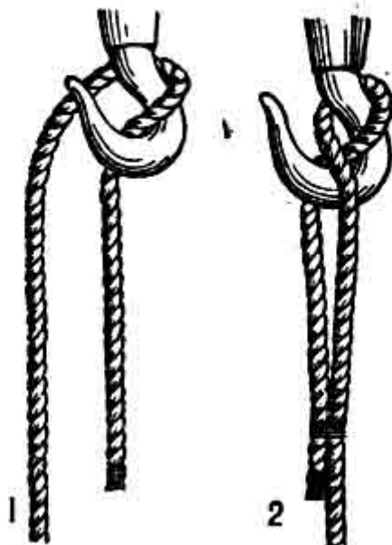
„Английская шнуровка“
