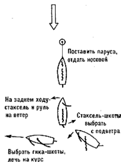
Рис. 123. Отход от бочки или причала на заднем ходу, когда за кормой есть место
