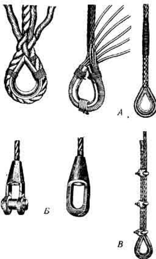
Рис. 68. Заделка концов такелажа:
