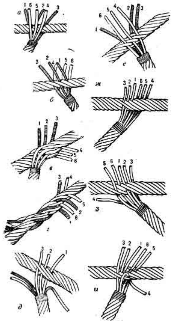
Рис. 67. Огон на стальном тросе
