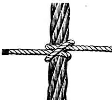
Выбленочный узел
