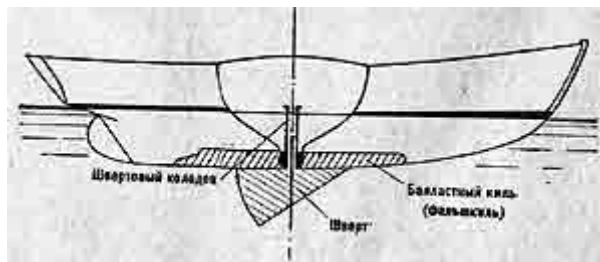
рис. 6. Яхта-компромисс
