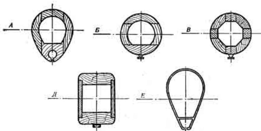
Рис. 37. Сечения рангоута:
