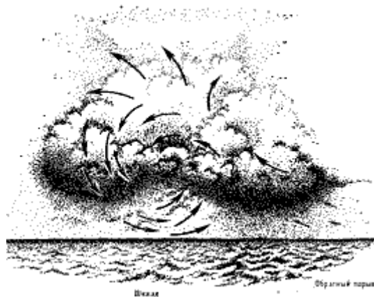
Рис 121 Схема циркуляции воздуха под шквальным облаком
