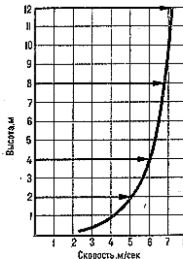
Рис. 89. Изменение скорости ветра с высотой
