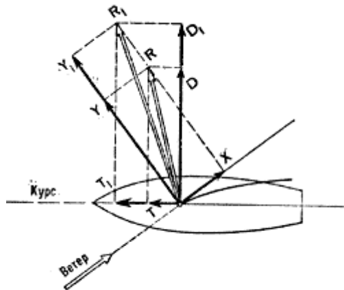
Рис. 95. Зависимость сил тяги и дрейфа от подъемной силы и лобового сопротивления паруса
