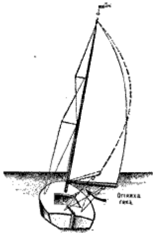
Рис. 112. «Закрутка» грота под ветер
