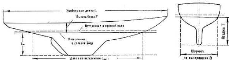
Рис. 76. Главные размерения килевой яхты
