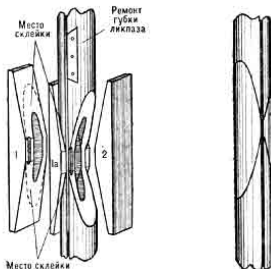
Рис. 74. Склеивание сломанной мачты
