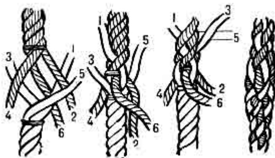
Рис. 63. Короткий сплесень на растительном тросе
