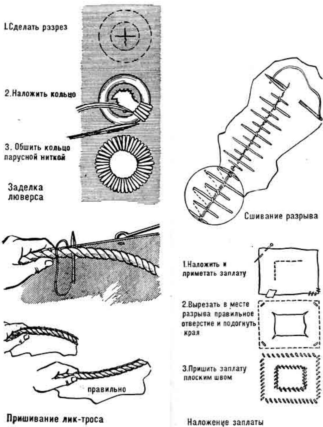
Рис. 72. Ремонт парусов
