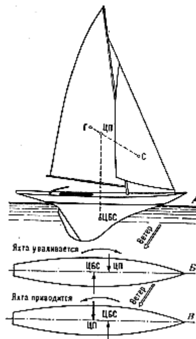
Рис. 99. Центровка яхты
