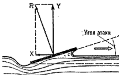
Рис. 87. Давление воды на движущуюся плоскую пластинку
