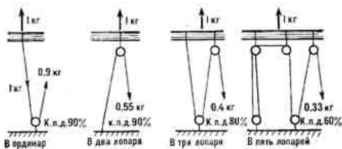
Рис. 44. Некоторые способы проводки гика-шкотов
