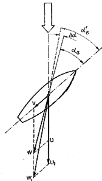
Рис. 92. В полосе сильного ветра можно идти круче
