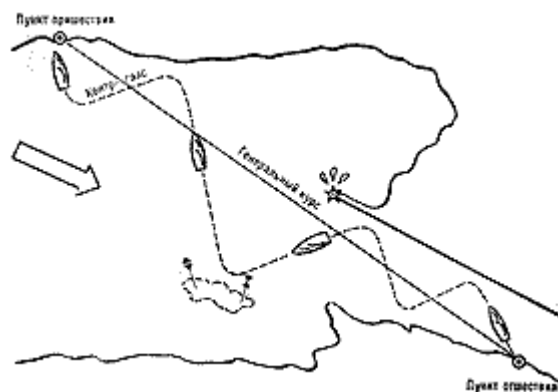
Рис. 107. Лавировка в узкости и в открытом бассейне
