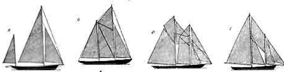
Рис. 15. Двухмачтовые яхты. А — бермудский иол; Б — стаксельный кэч. В — гафельная шхуна; Г — бермудская стаксельная шхуна
