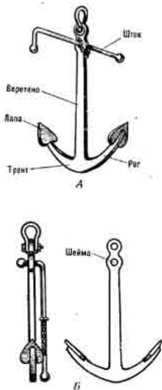
Рис. 52. Адмиралтейский якорь и его части
