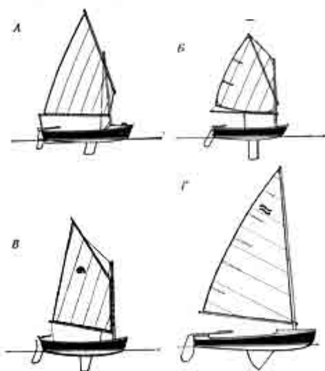
Рис. 12. Кэты:
