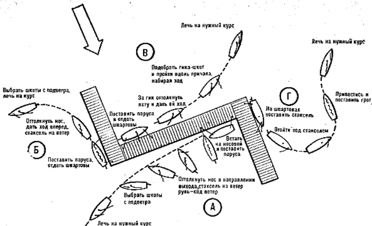
Рис. 124. Как отойти от причала:
