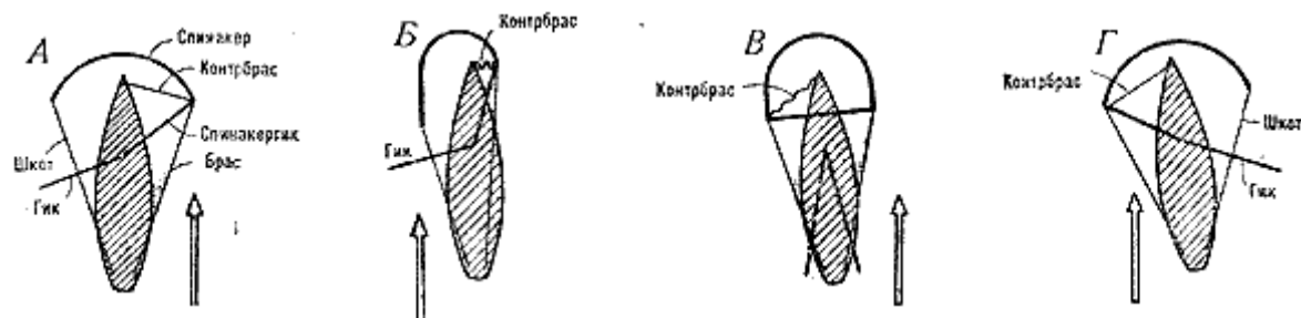
Рис. 115. Поворот через фордевинд со спинакером
