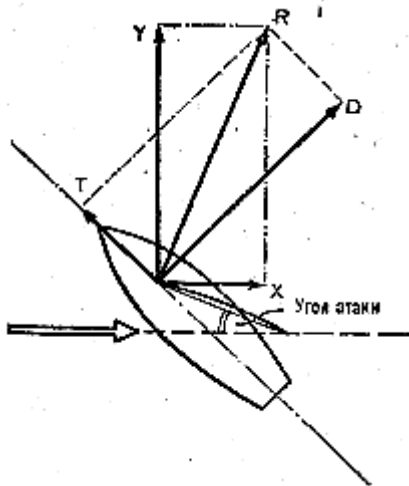
Рис. 94. Силы, действующие на паруса яхты
