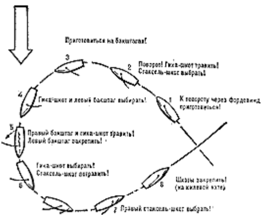
Рис. 110. Поворот через фордевинд
