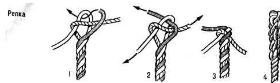
Рис. 68. Заделка концов такелажа:
