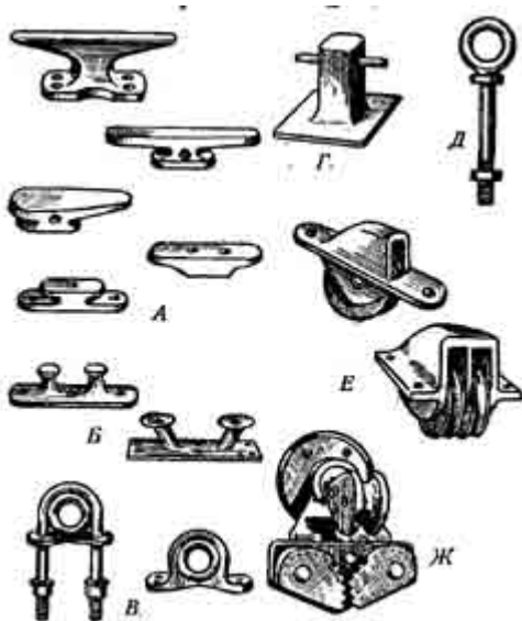
Рис. 50. Дельные вещи:
