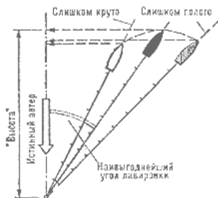
Рис. 106. Наивыгоднейший курс при лавировке. Несмотря на то что белая яхта идет круче, а полосатая быстрее, черная имеет наибольшую скорость лавировки
