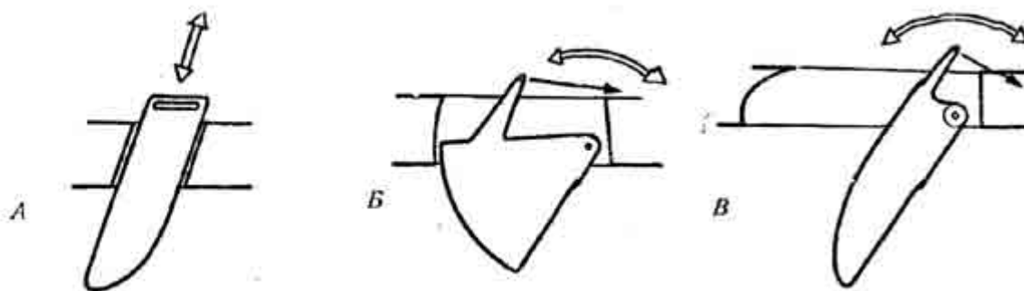
Рис. 33. Типы швертов:
