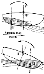
Рис. 79. Остойчивость швертбота на волне
