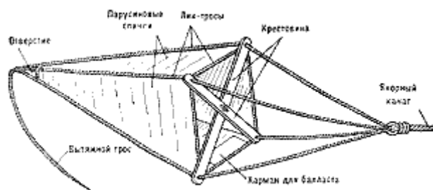
Рис. 117. Плавучий якорь
