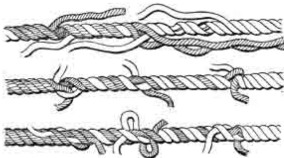
Рис. 64. Лонгоспесень (длинный сплесень)
