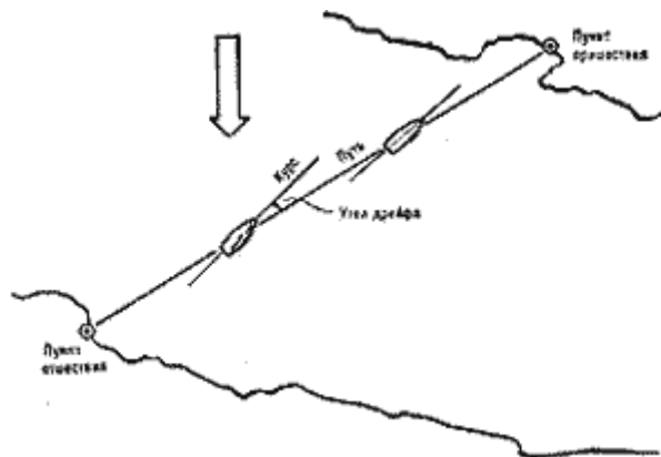
Рис. 105. Плавание курсом бейдевинд
