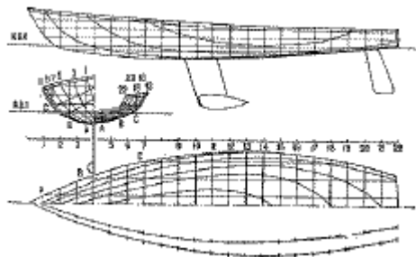
Рис. 85. Теоретический чертеж килевой яхты класса «Темпест»
