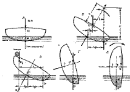
Рис. 78. Остойчивость швертбота
