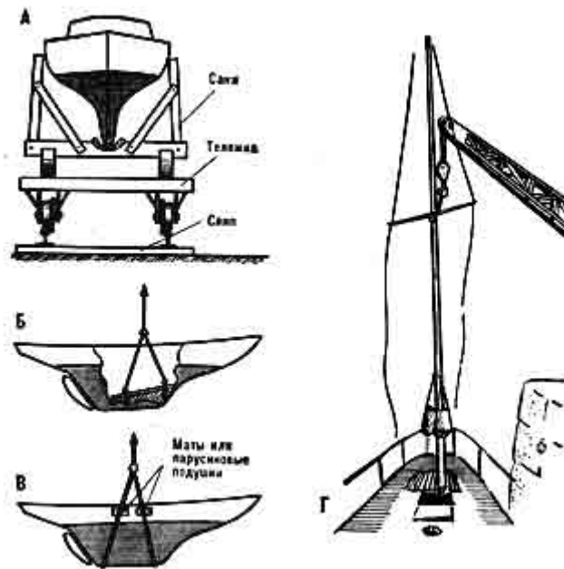
Рис. 75. Способы подъема и спуска яхты:
