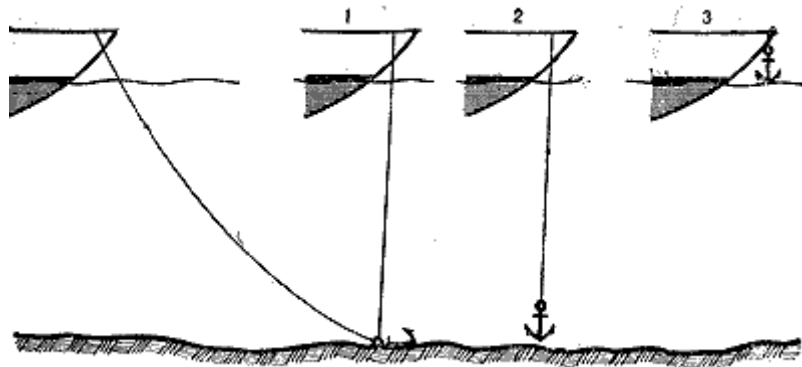
Рис. 127. Схема съемки с якоря: 1— «панер»; 2— «якорь встал»; 3 — «якорь чист»
