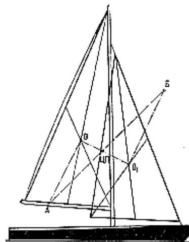
Рис. 98. Графический способ нахождения центра парусности
