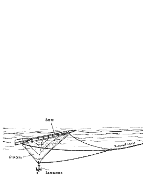
Рис. 119. Временный плавучий якорь
