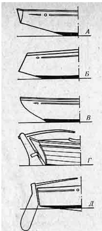
Рис. 10. Формы кормовых частей:
