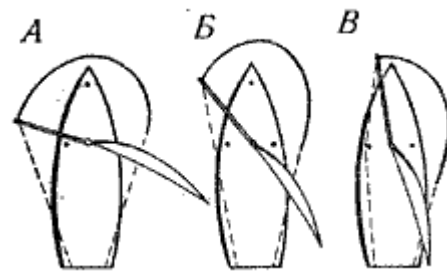
Рис. 114. Схема несения спинакера на разных курсах А — на фордевинде, Б — в бакштаг, В — в галфвинд
