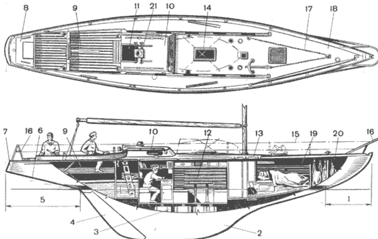
Рис.1: Килевая яхта и ее части: 1-носовой свес; 2-плавник и фальшкиль; 3-трюм; 4-перо руля; 5-кормовой свес; 6-подзор; 7-транец; 8-ют; 9-кокпит; 10- рубка; 11-входной люк; 12-каюта; 13-палуба; 14-светлый (световой) люк; 15-леерное ограждение; 16-носовой и кормовой релинги; 17- якорное устойство (якорь, цепь, битенг, палубный клюз); 18-бак; 19-кубрик; 20-форпик; 21-компас.
